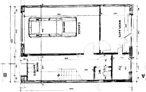
GELIJKVLOERS
