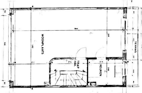
1 VERDIEPING
